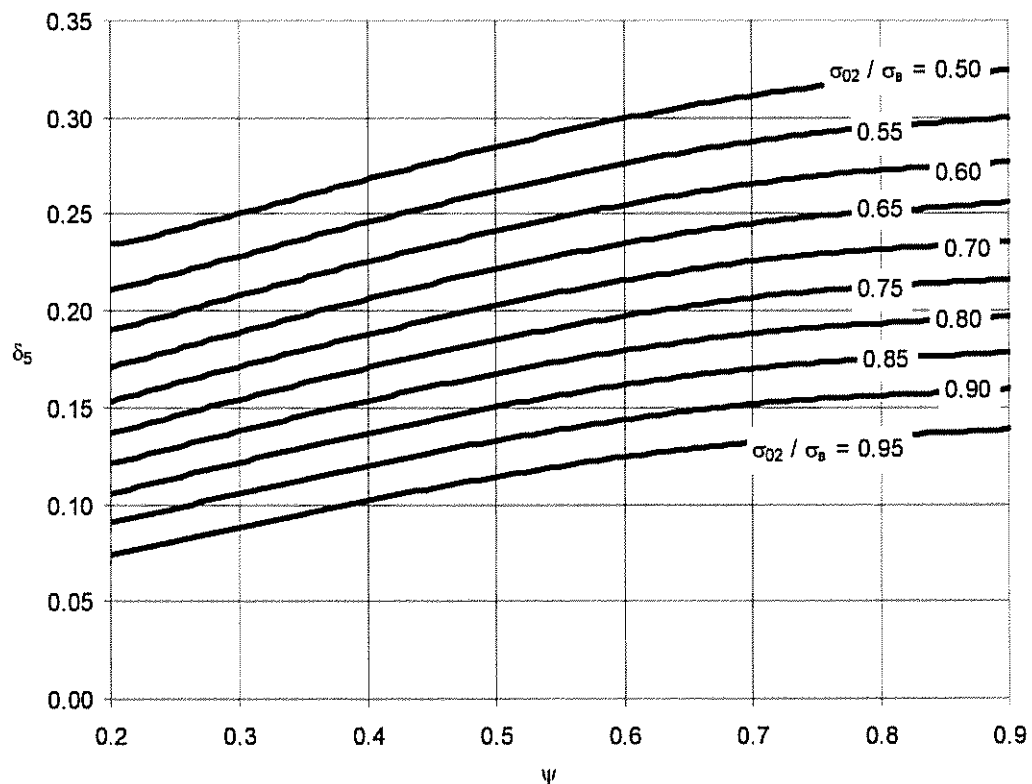
Рисунок 4. Определение относительного сужения после разрыва \psi
