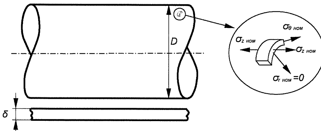
Рисунок 3. Схема нагружения секции трубы
