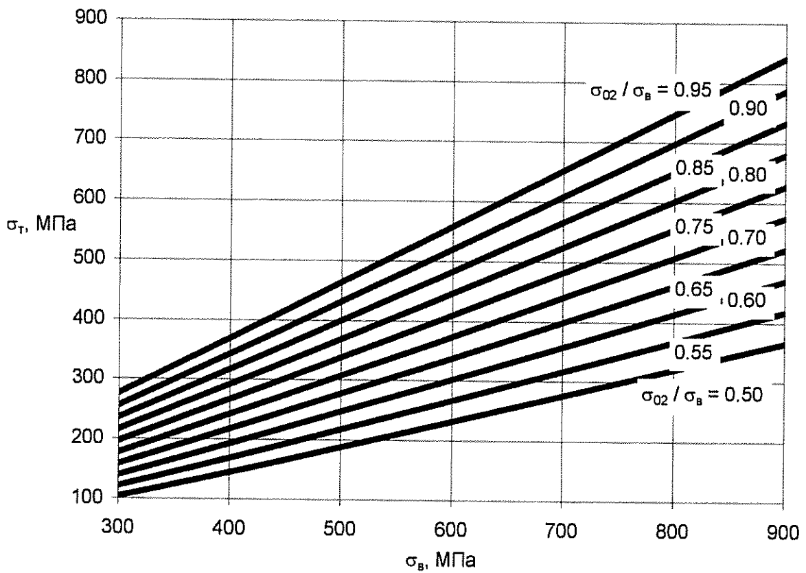
Рисунок 6. Определение предела текучести \sigma_T
