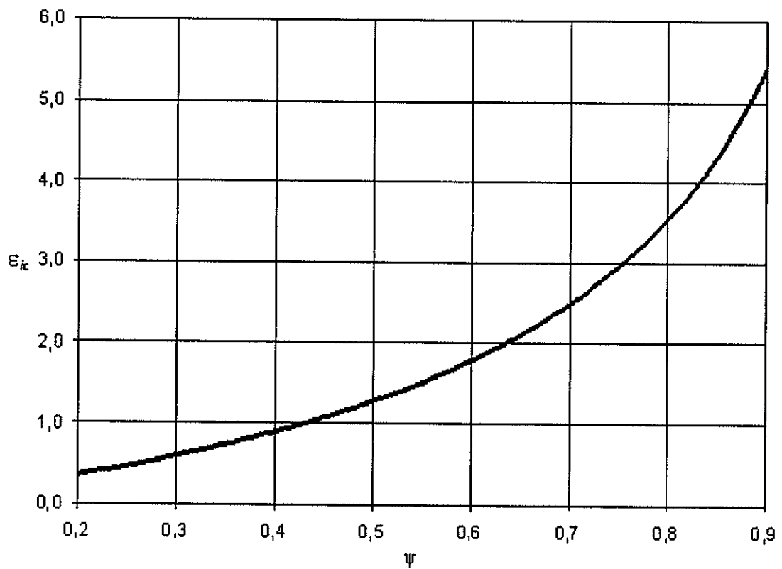
Рисунок 8. Определение разрушающей интенсивности деформации \varepsilon_{0c}
