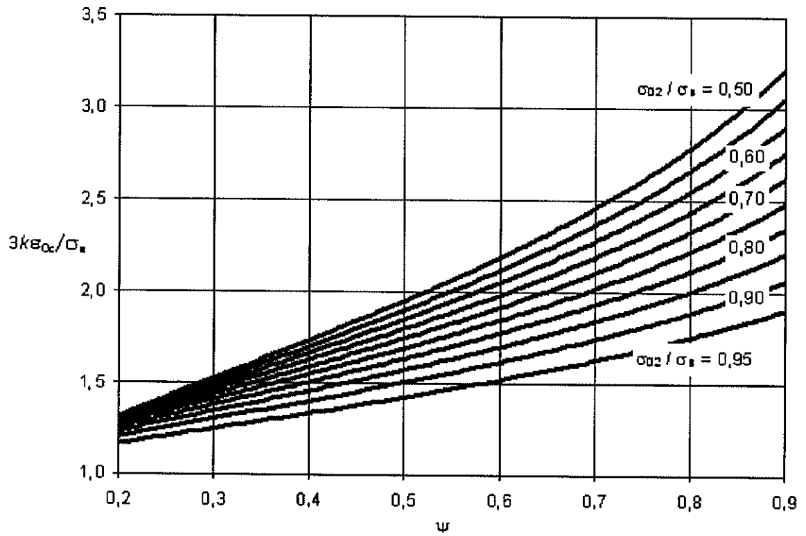
Рисунок 7. Определение разрушающей объемной деформации \varepsilon_{0c}
