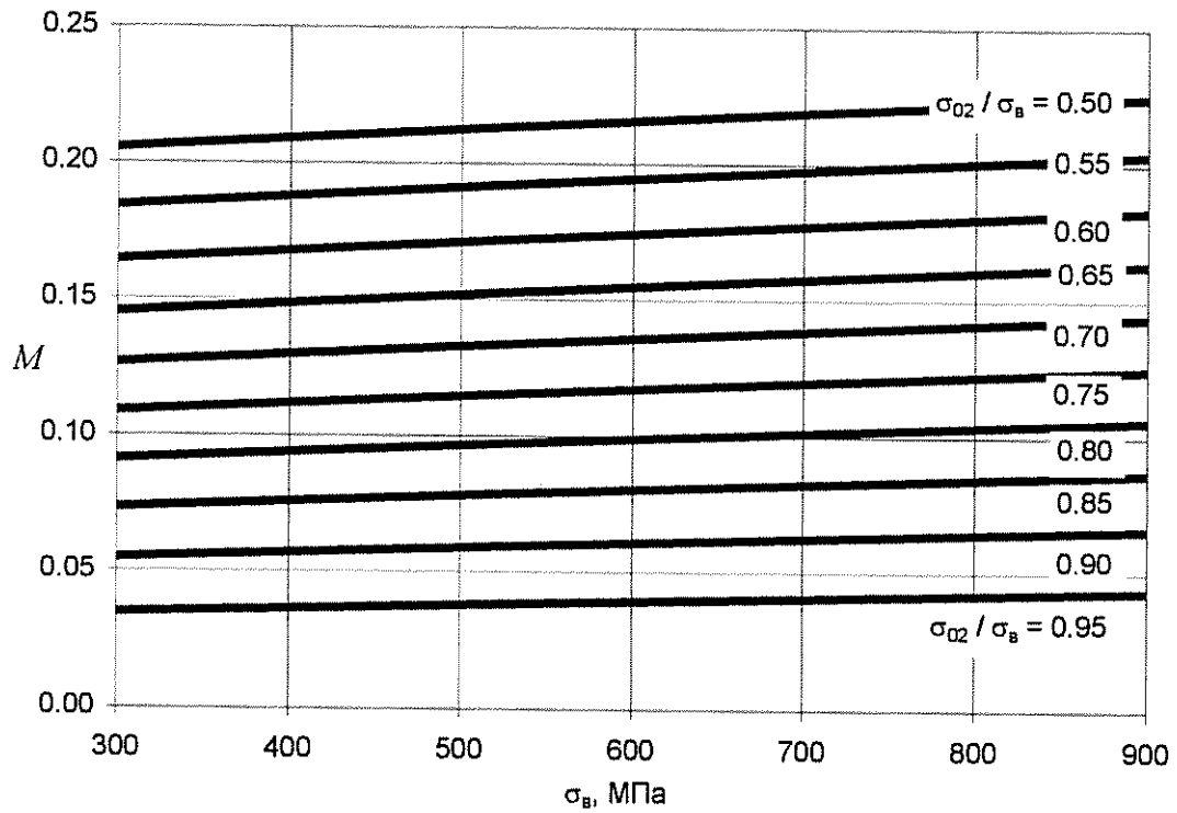
Рисунок 5. Определение коэффициента деформационного упрочнения M
