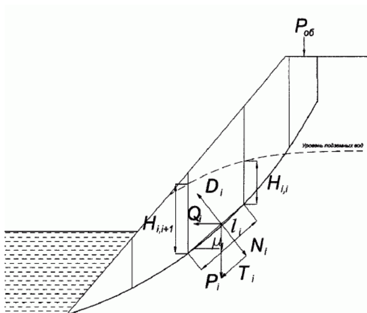
Рисунок 2. Расчет устойчивости обводненного изотропного откоса с учетом воздействия сейсмических сил методом алгебраического сложения сил
