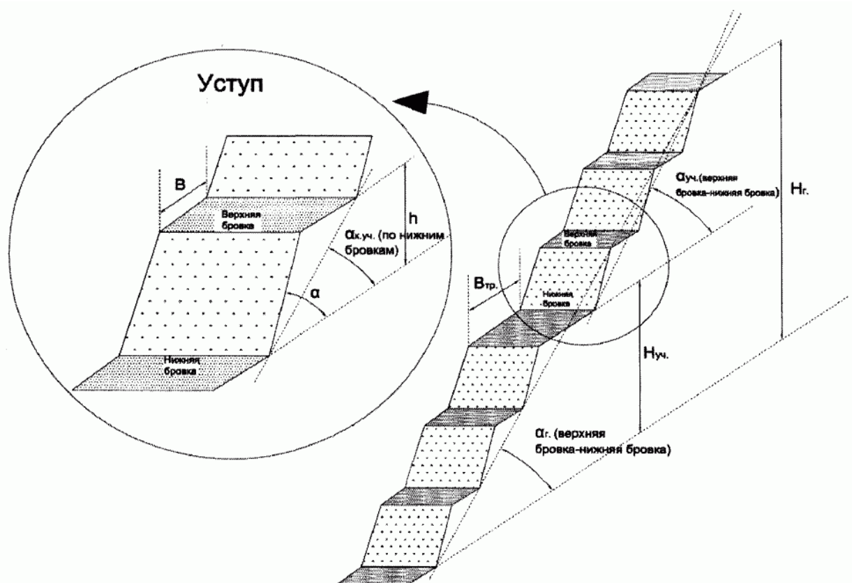
Рисунок 1. Схема конструкции бортов и уступов: h, Н уч , Н г - соответственно высота уступа, групп уступов, борта; α, α уч , α к.уч , α г - соответственно, угол откоса уступа, угол откоса группы уступов, конструктивный угол откоса группы уступов и угол откоса борта карьера, разреза; В, В тр - соответственно, ширина предохранительной и транспортной бермы
