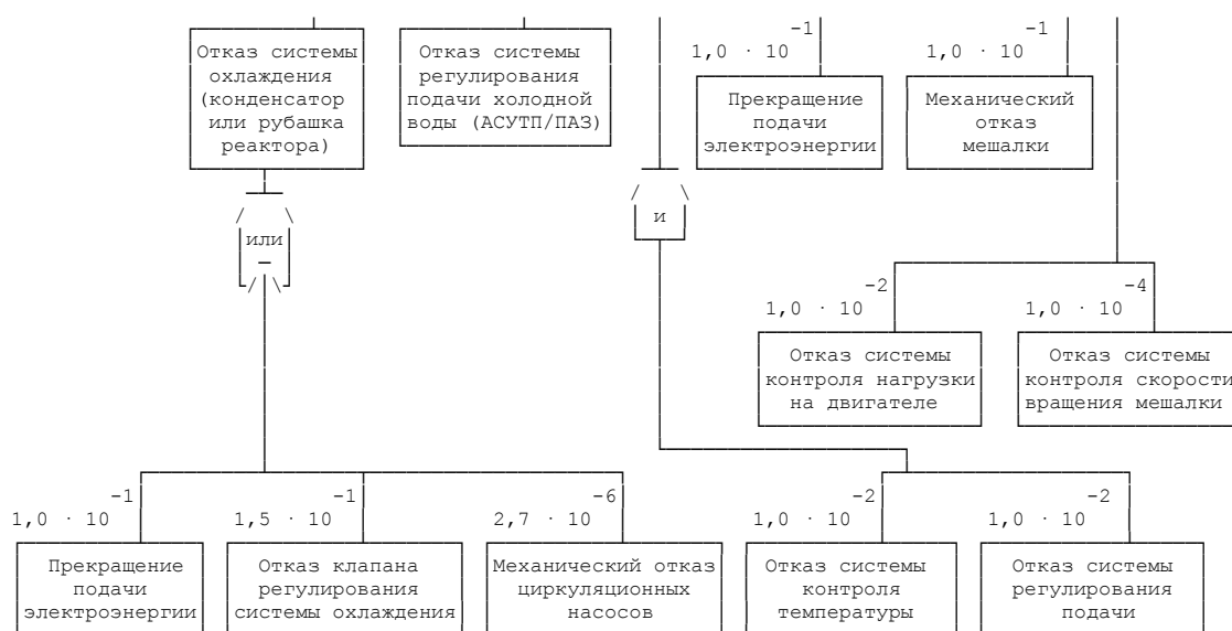
Рисунок 8-1. Пример дерева отказов для химических реакторов
