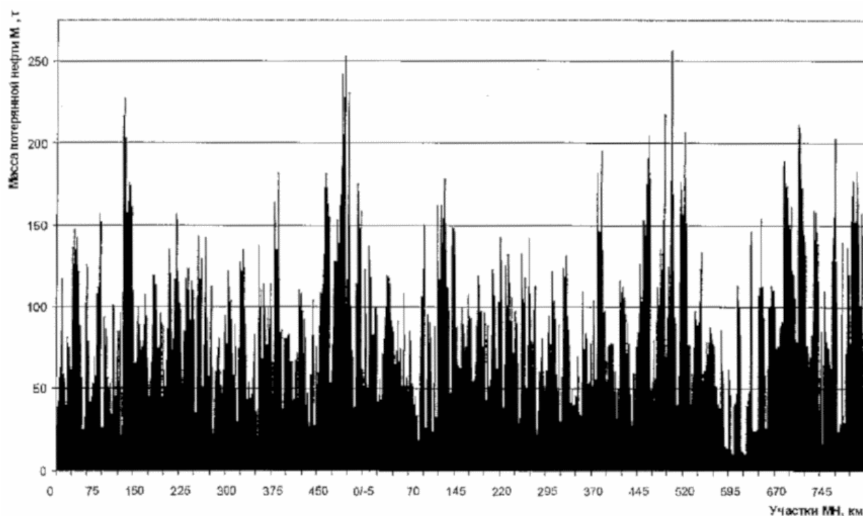
Рисунок 8-3. Пример распределения показателей риска по трассе магистрального нефтепровода (км) и ранжирования ОПО
